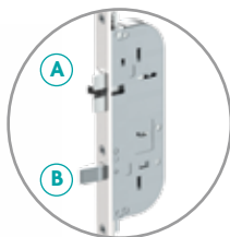
A 3 PÊNES 1/2 TOUR à archet facilitant l'entrée et la prise dans la gâche centrale.
