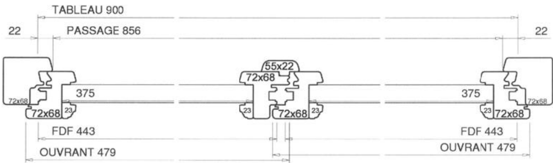
Coupe horizontale OF 2 dormant de base, battement central standard
