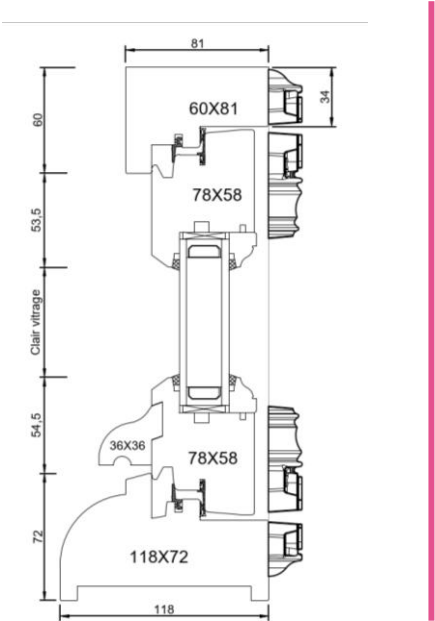
Coupe verticale OF1 & OF2 dormant de base
